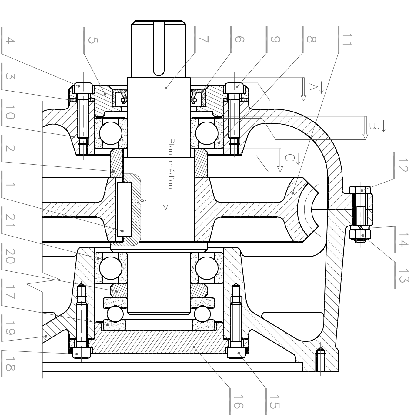
Réducteur roue et vis sans fin
