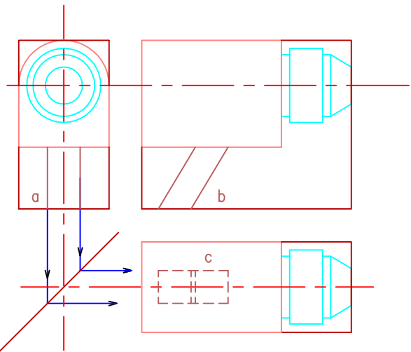
4- Dessin de la poignée
